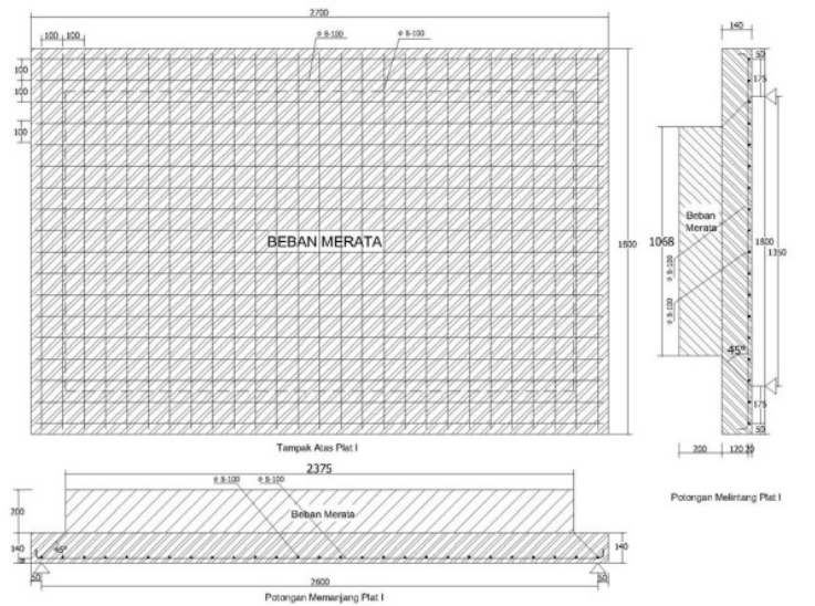
Gambar 4. Pelat pejal (PP)
