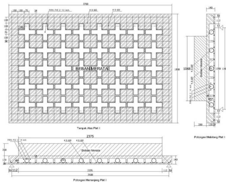
Gambar 5. Pelat berongga tebal 14 cm (PB-1)
