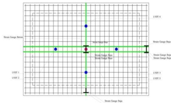
Gambar 8. Perletakan strain gauge dan LVDT
