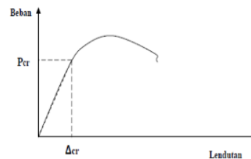
Gambar 3. Kurva beban terhadap lendutan
