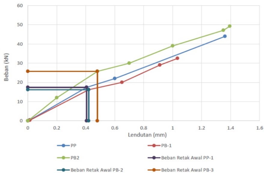
Gambar 10. Hubungan beban dan lendutan pada retak awal
