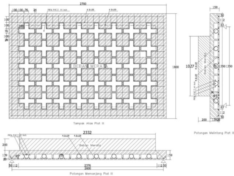
Gambar 6. Pelat berongga tebal 15,9 cm (PB-2)
